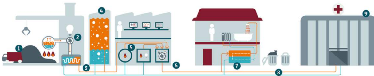
Impianto di teleriscaldamento, Bolzano
